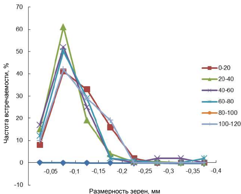
Рисунок 1. Совмещенные графики гранулометрического состава золота на различных глубинах развития гипогенно-гипергенной минерализации Гумешевского месторождения. Справа – интервалы глубины отprobования в метрах. Figure 1. Combined graphs of the granulometric composition of gold at various depths of development of hypogene-supergene mineralization of the Gumeshevskoye deposit. To the right – intervals of depth of sampling in meters.
