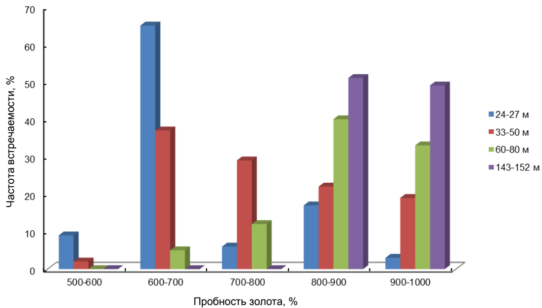
Рисунок 4. Изменение пробности золота из гипогенно-гипергенных руд месторождения с глубиной. Figure 4. Change in the fineness of the gold from the hypogene-supergene ores of the deposit with depth.
