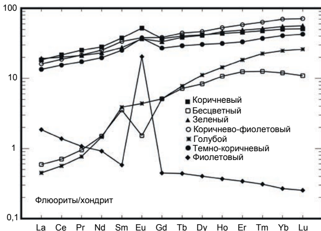
Рисунок 4. Распределение нормированных по хондриту редкометалльных элементов во флюоритах Мариинского месторождения.
