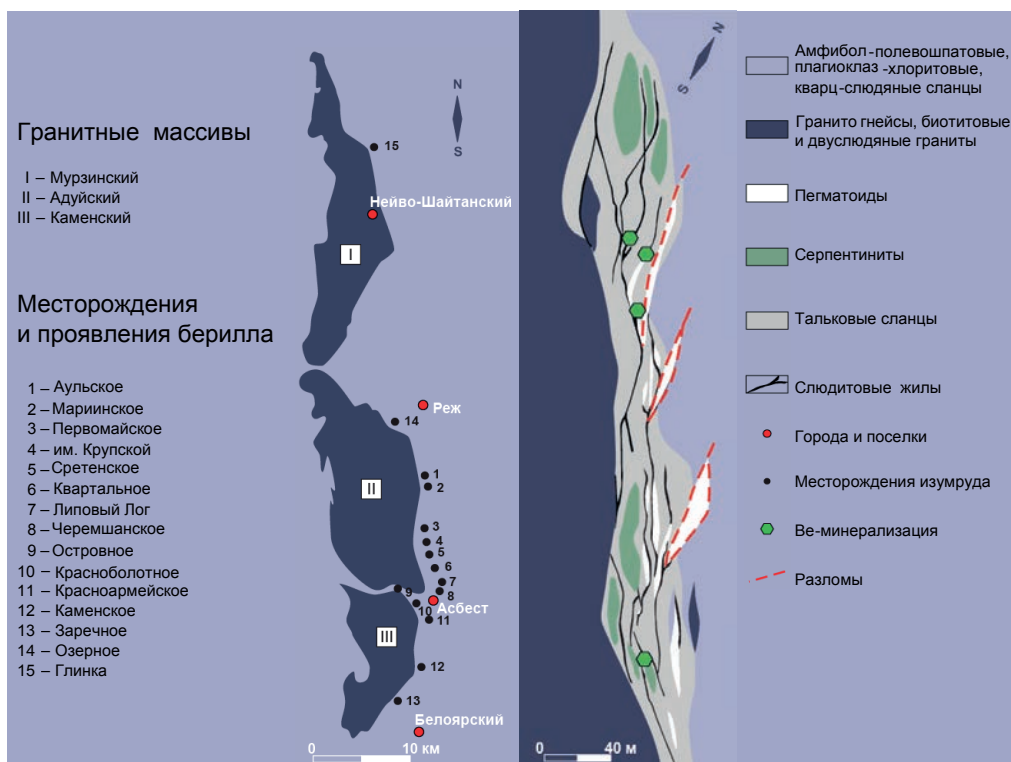
Рисунок 1. Схема размещения месторождений и проявлений берилла и самоцветов (изумруд, александрит) в пределах Мурзинско-Адуйской самоцветной субпровинции.
